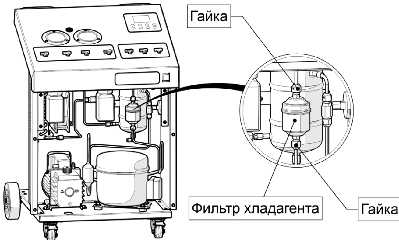
Рис. 10 Замена фильтра хладагента
