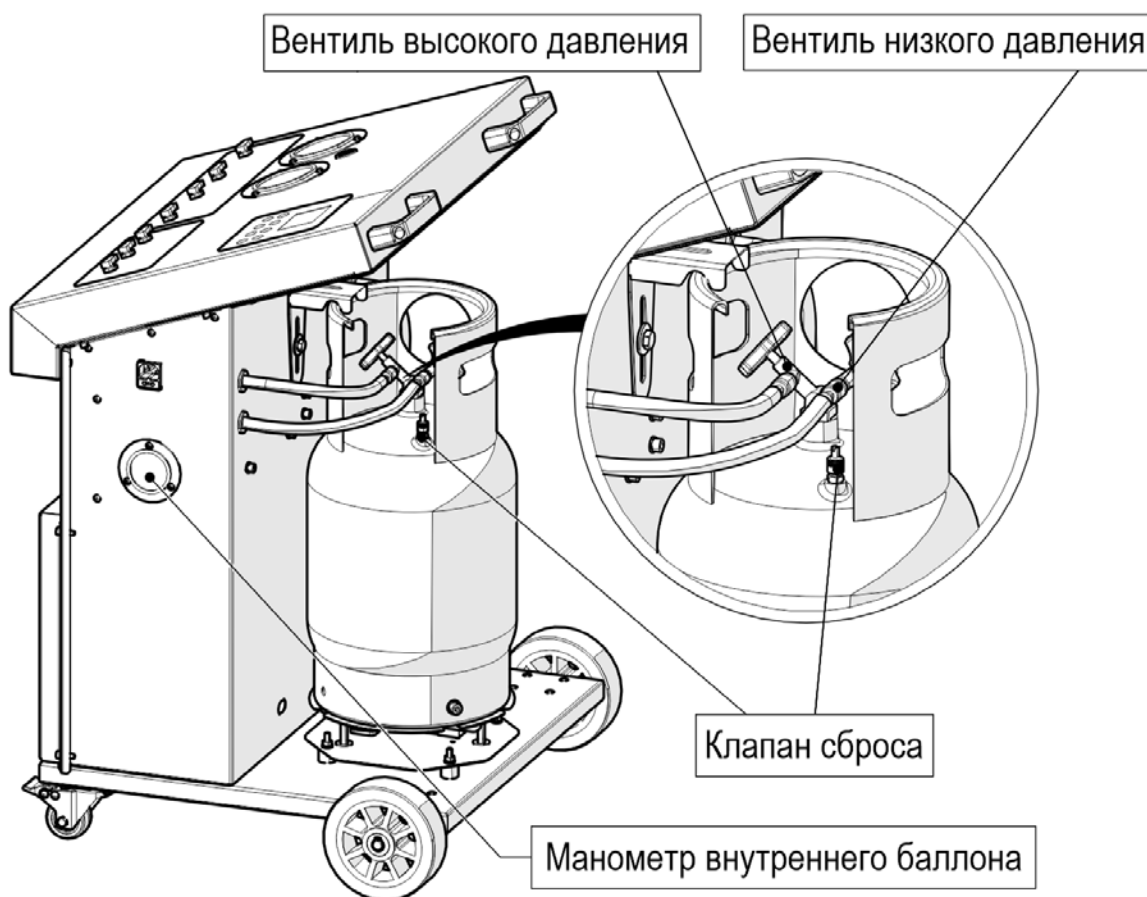
Рис. 8 Сброс неконденсируемых газов
