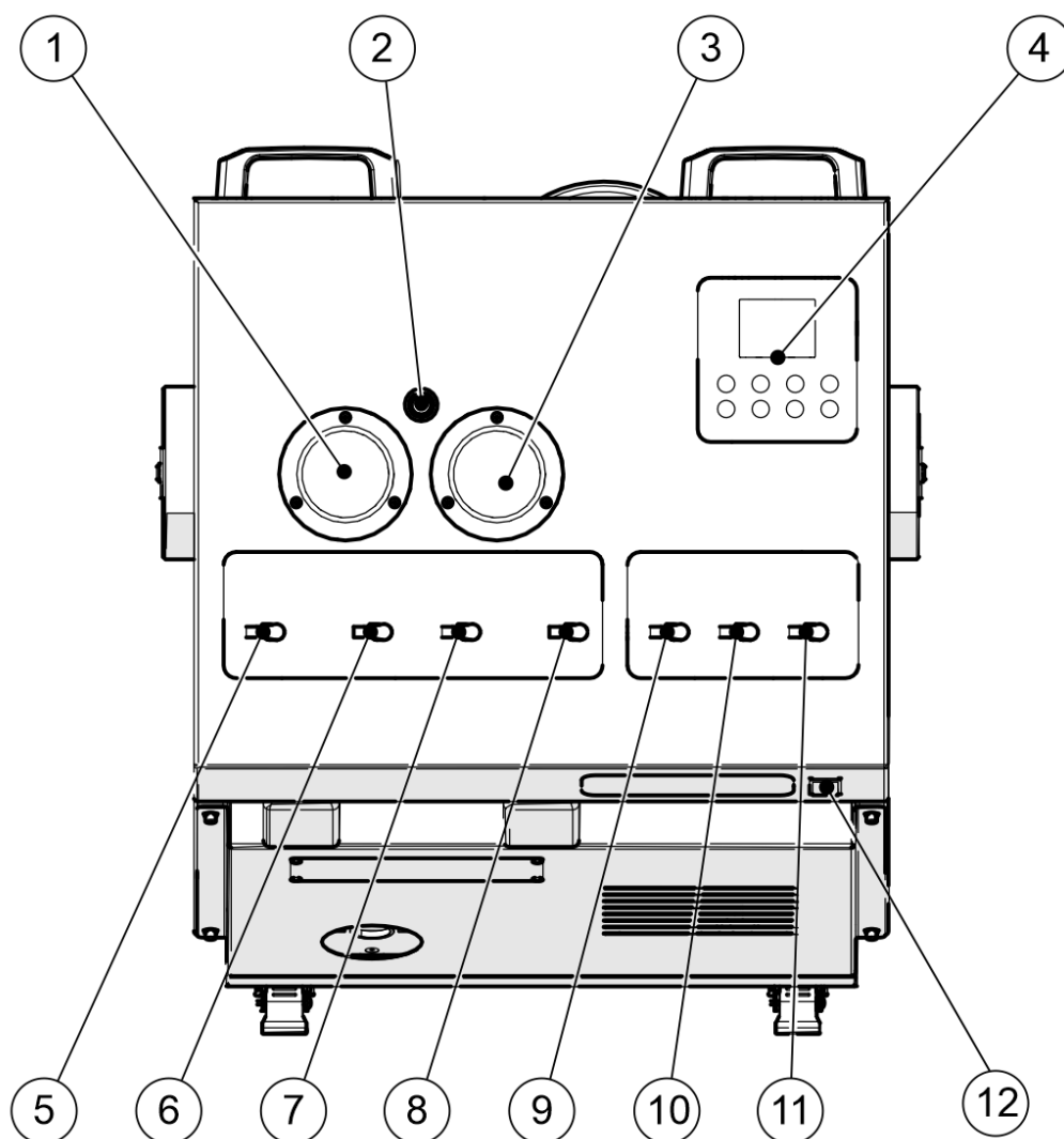
Рис. 3 Лицевая панель ODA-250
