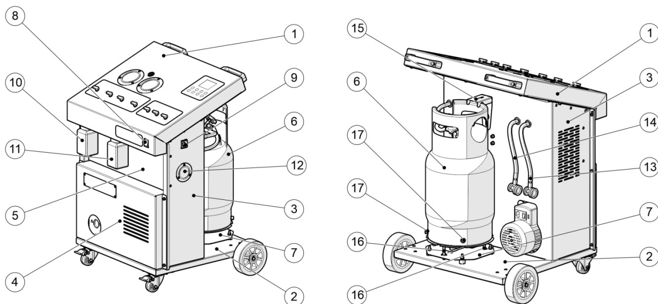
Рис. 2 Основные элементы станции ODA-250
