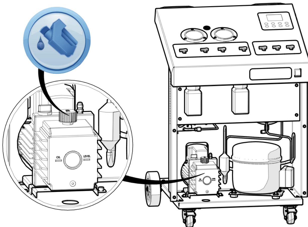
Рис.9 Заправка вакуумного насоса
